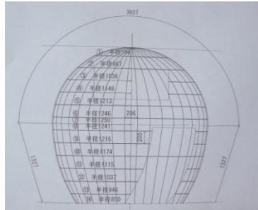
骨組鉄筋の図面設計
